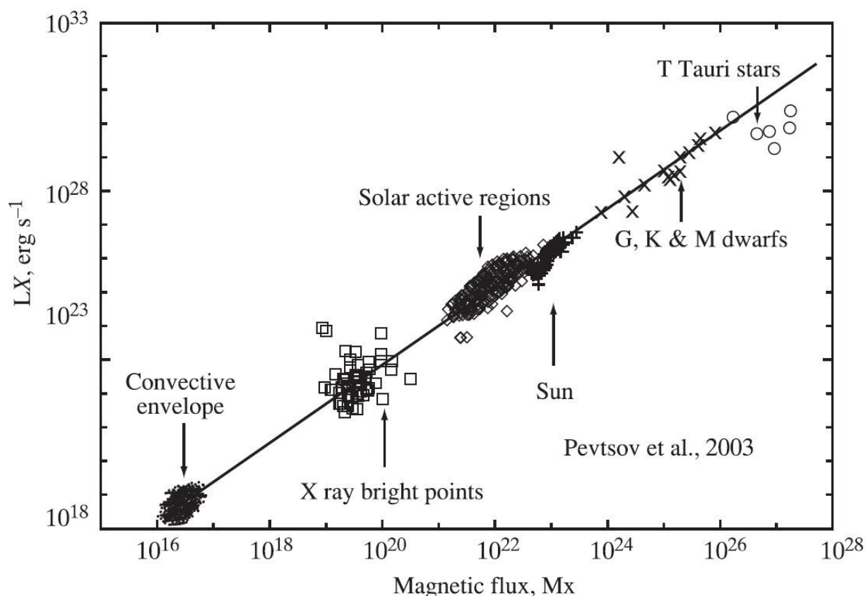
Рис. 2. Зависимость потока мягкого рентгеновского излучения в динамике (0,3–4,4 кэВ) от величины магнитного потока для Солнца и звёзд
