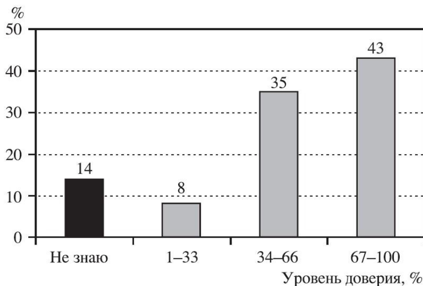
Рис. 5. Уровень доверия научным знаниям о Вселенной.
